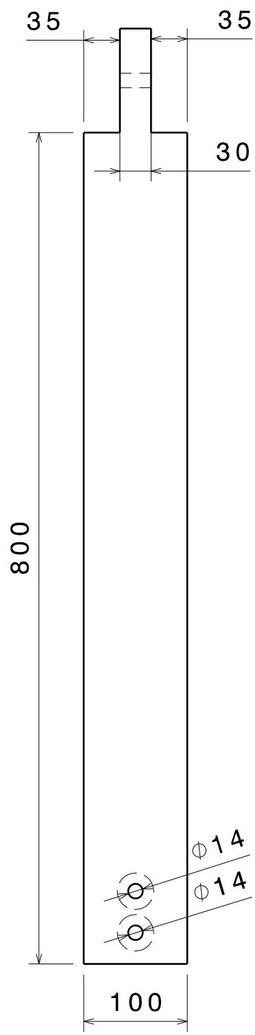
Vorderansicht
