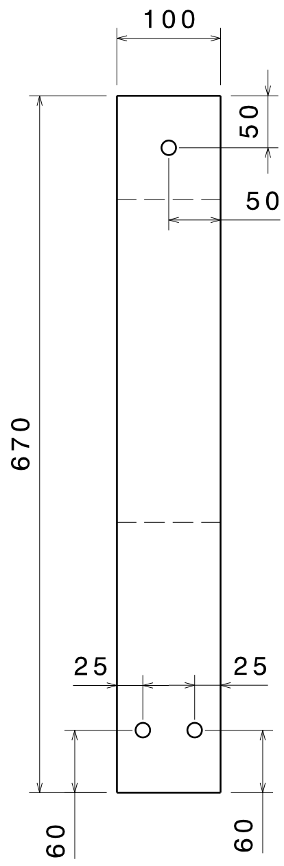
Seitenansicht rechts
